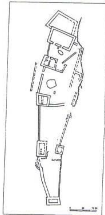
איור (163): מבצר תפן. תוכנית האתר. (באדיבות ד"ר ר. פרנקל ומר. נצוב).
