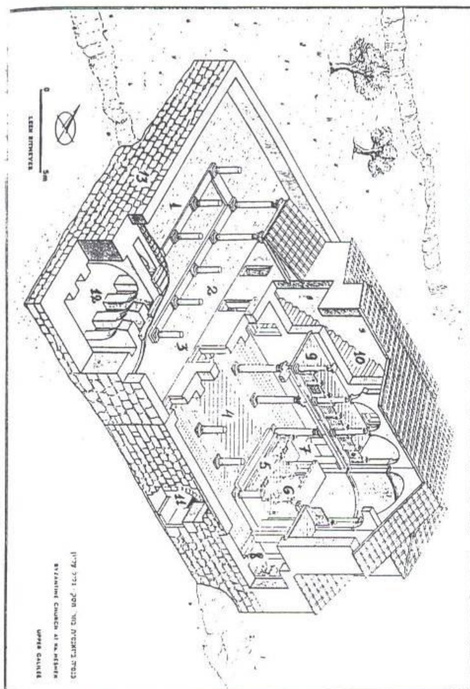
איור (165): כנסיית סנט ג'ורג' בחורבת חֶשֶק, שהוזר האתר (כאדיבות מר מרדכי אביעם). 1. האטריום, 2. הנרתיקס, 3. כניסה ראשית, 4. האולם המרכזי, 5. הבימה, 6. האפסיס המרכזי, 7. האפסיס הצפוני, 8. האפסיס הדרומי, 9. הקומה השנייה, 10. גרם מדרגות אשר הוביל אל הקומה השנייה, 11. הקריפטה, 12. מאגר המים, 13. חומת-הגדר.
