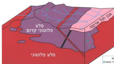
לאחר הפסקה ארוכה המשך ההשקעה היבשתית הקדומה (100-130 מיליון שנים)
