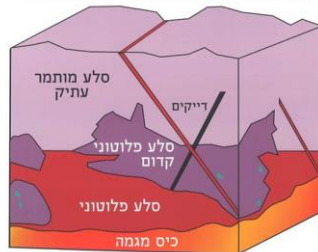
השלב המגמטי הקדום (לפני 580-630 מיליון שנים)
