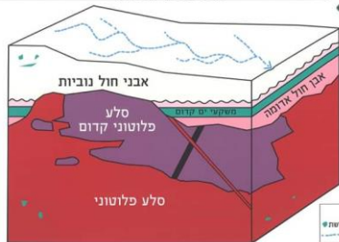
לאחר הפסקה ארוכה המשך ההשקעה היבשתית הקדומה (100-130 מיליון שנים)
