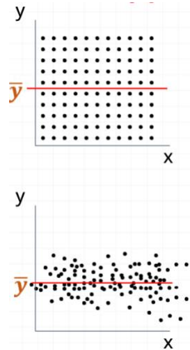
אין קשר לינארי
