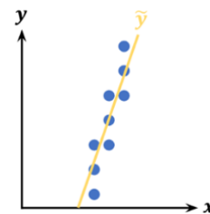
פיזור אופקי קטן S_x קטנה m גדול
