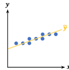
פיזור אנכי קטן S_y קטנה m קטן
