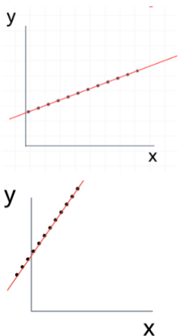
קשר לינארי מושלם
