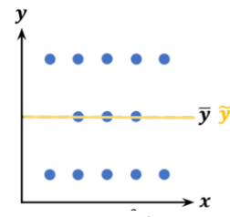
קו הרגרסיה מתלכד עם קו הממוצע \bar{y} m = 0
