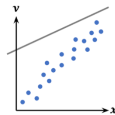
ברור שהקו לא יעבור כאן...
