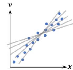
הוא יעבור בצורה כלשהי במרכז ענן התצפיות
