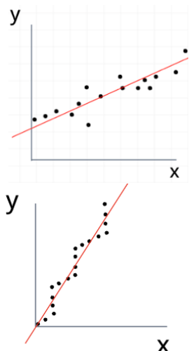
קשר לינארי לא מושלם
