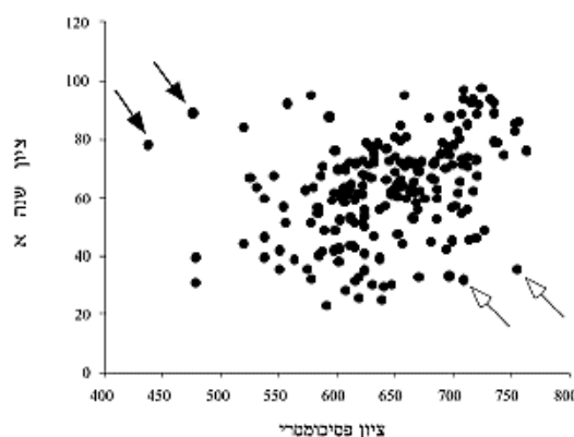
איור 3. דיאגרמת פיזור של תלמידי מתמטיקה לפי הציון הפסיכומטרי וציון שנה א באוניברסיטה
