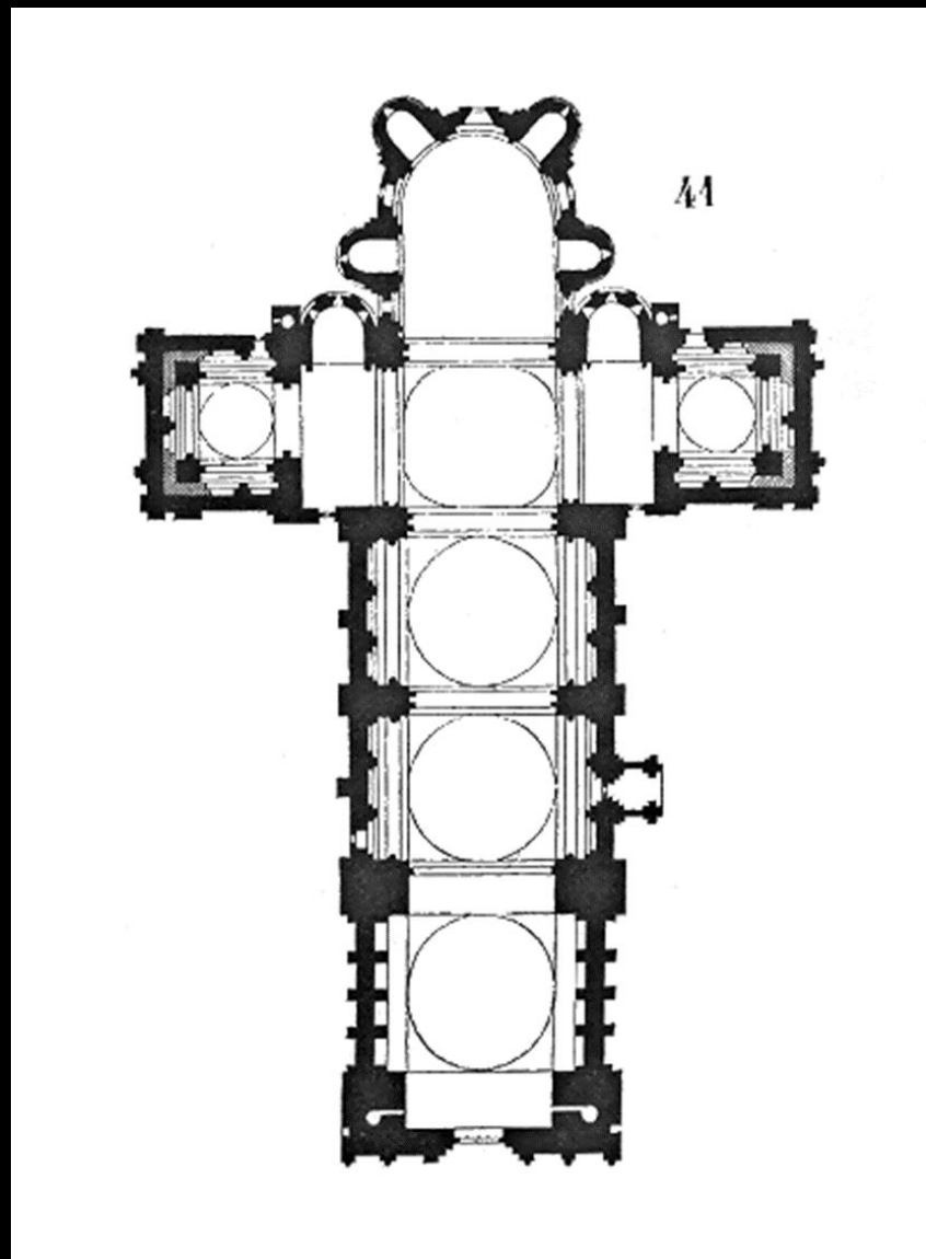
תכניות מבנה קתדרלת אנגולם לעומת קתדרלת שארטר
