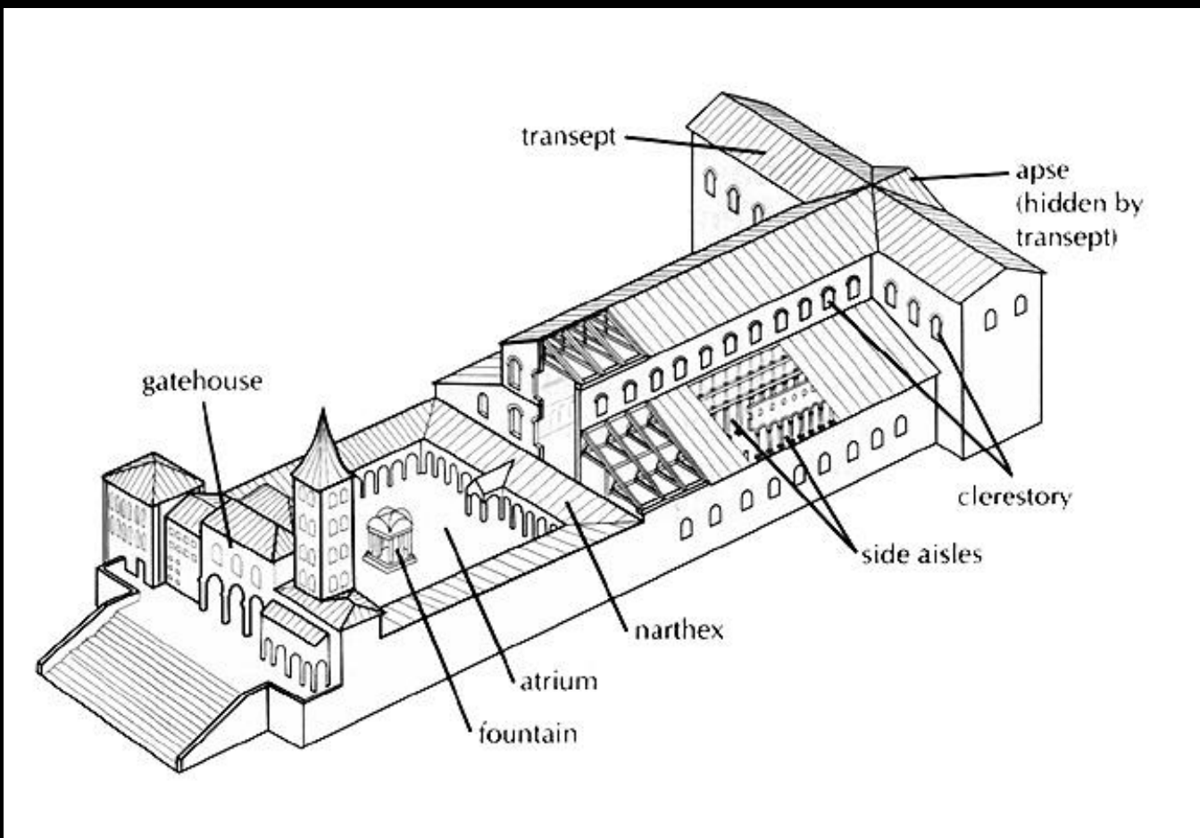
בזיליקת ס. פטרוס, (S. Pietro), שחזור, מאה 4, 30X100 מ', רומא.
