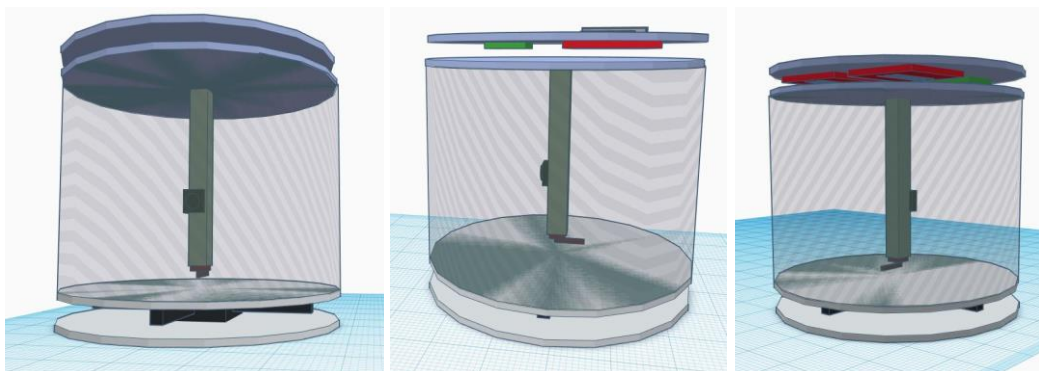
מודל תלת מימדי של המערכת משלושה כיוונים שונים בתוכנת מידול ממוחשבת.
