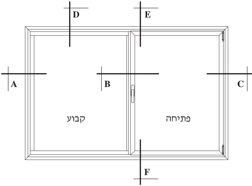
מבט פנים סוג הפתיחה של החלון:
