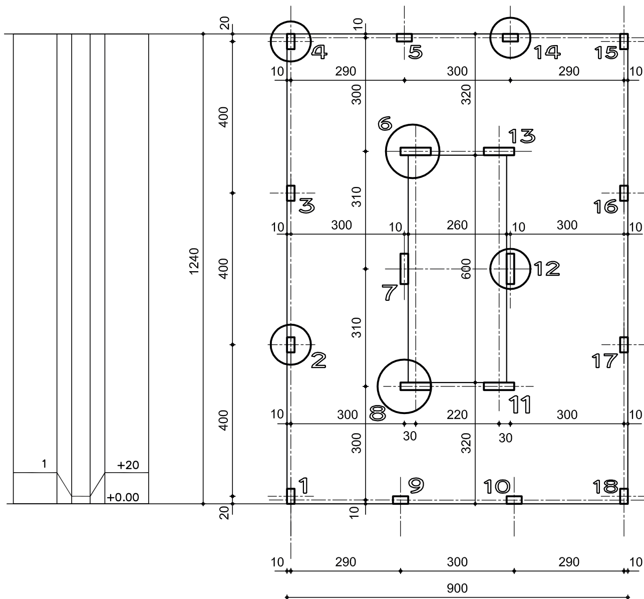
תוכנית, קנ"מ 1:100
