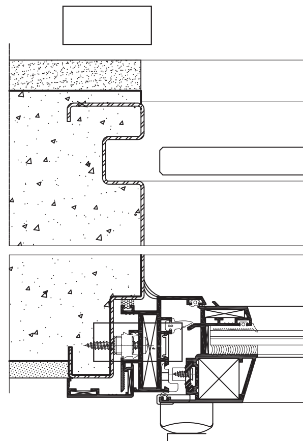
פרט A
