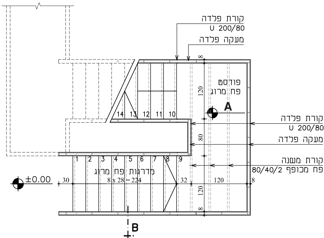
תכנית מדרגות פלדה, קנ"מ 1:50
