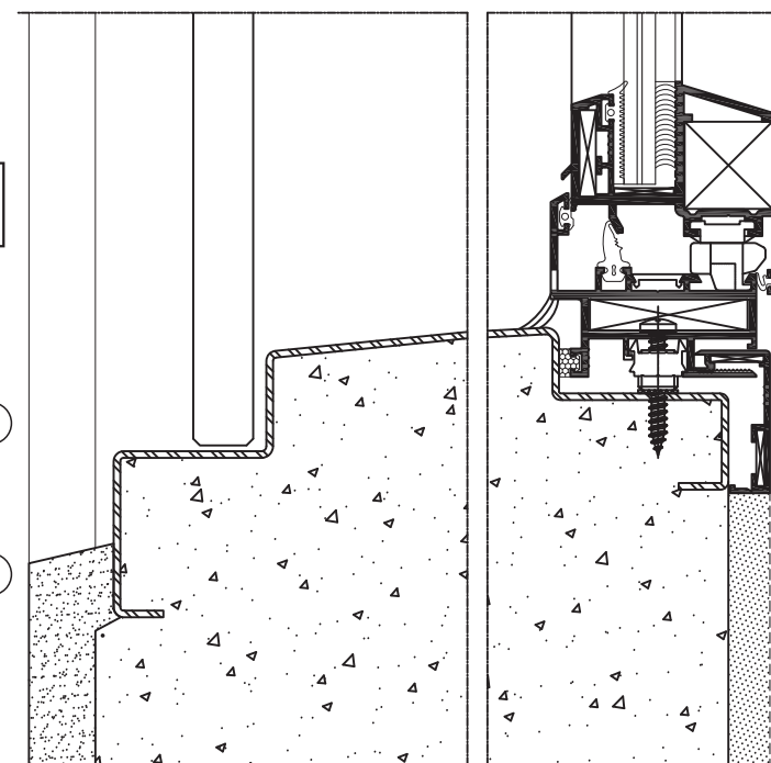
פרט D
