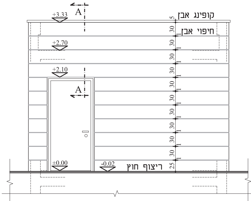
חזית, קנ"מ 1:50
