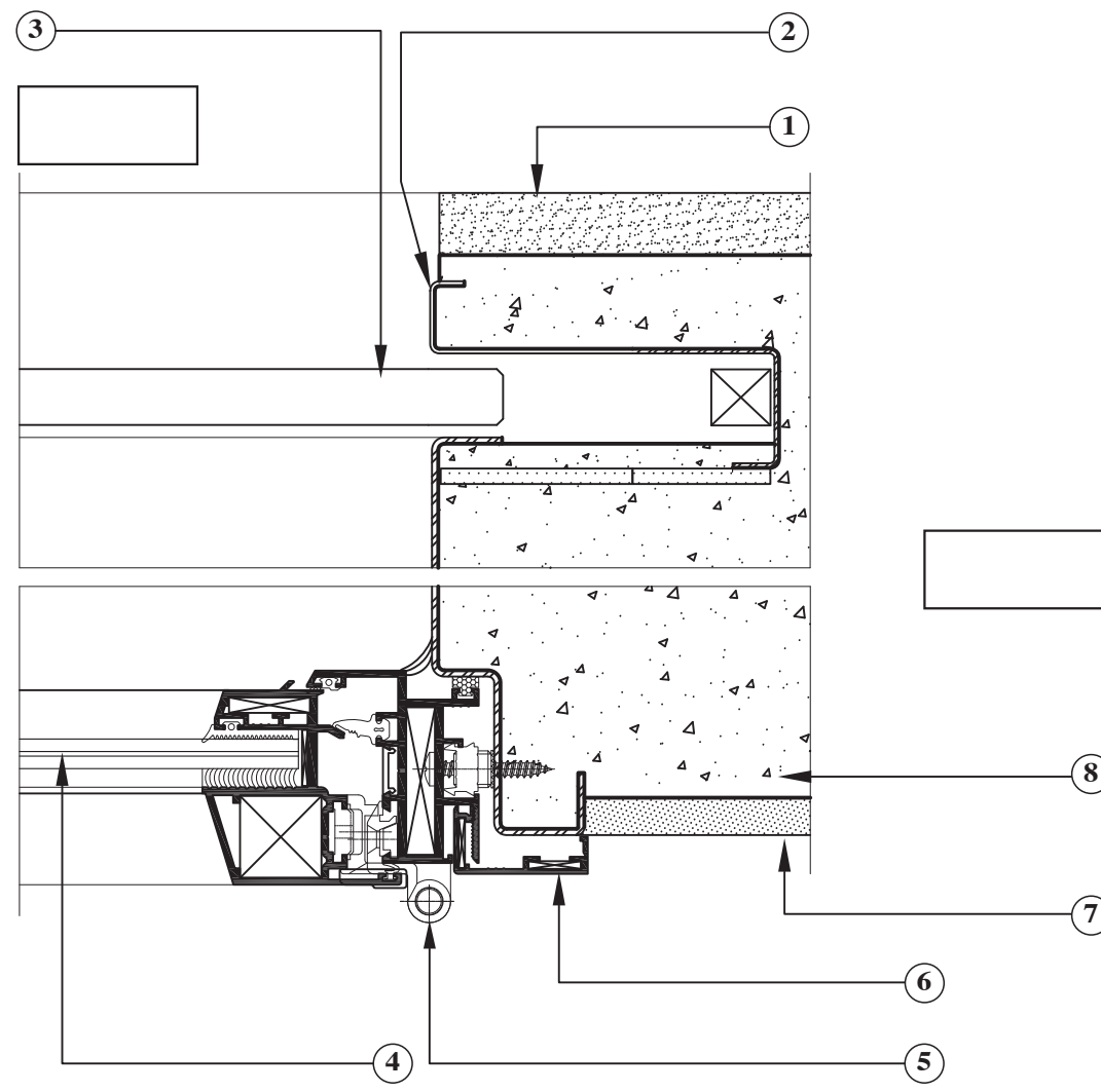
פרט B
